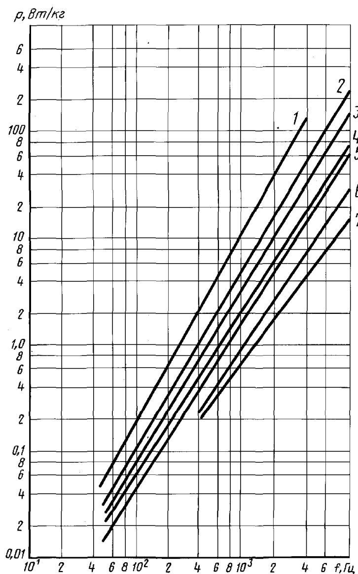
Зависимость P_{0,5} от частоты для сплавов марок: 1 — 79НМ и 80НХС толщиной 0,35 мм; 2 — 79НМ толщиной 0,2 мм; 3 — 80НХС толщиной 0,2 мм; 4 — 79НМ толщиной 0,1 мм; 5 — 80НХС толщиной 0,1 мм; 6 — 79НМ и 80НХС толщиной 0,05 мм; 7 — 79НМ толщиной 0,2 мм
