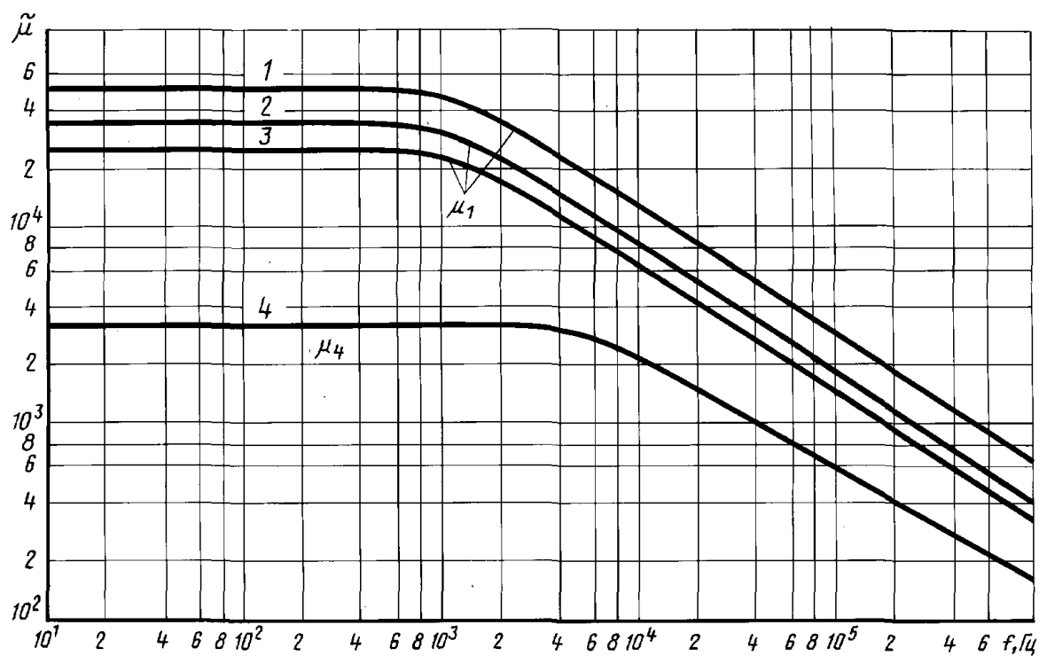
Зависимость \tilde{\mu} от частоты для сплавов в лентах толщиной 0,1 мм марок: 1 — 81НМА и 83НФ; 2 — 80НХС; 3 — 79НМ; 4 — 50Н
