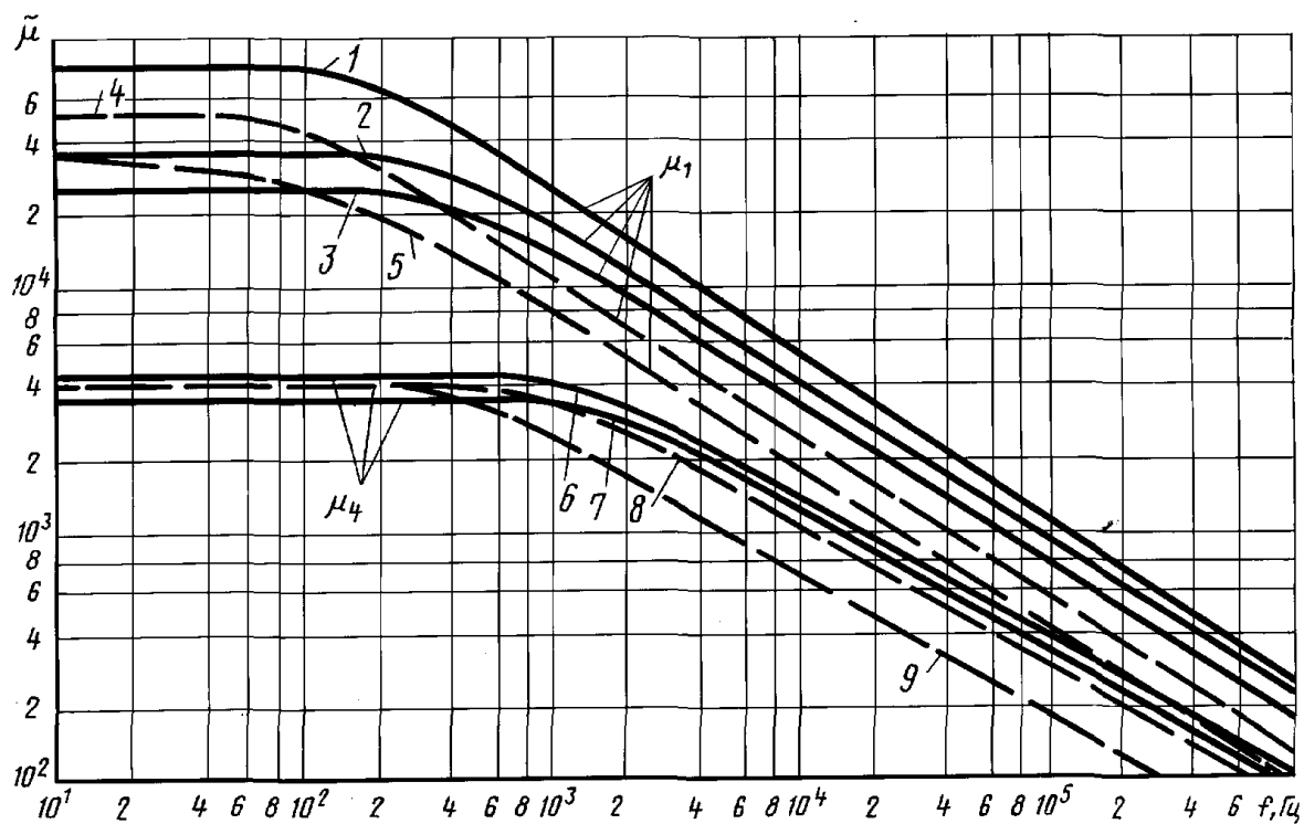
Зависимость \tilde{\mu} от частоты для сплавов марок: 1 — 81НМА толщиной 0,2 мм; 2 — 80НХС толщиной 0,2 мм; 3 — 79НМ толщиной 0,2 мм; 4 — 80НХС толщиной 0,35 мм; 5 — 79НМ толщиной 0,35 мм; 6 — 50НХС толщиной 0,2 мм; 7 — 50НМ толщиной 0,2 мм; 8 — 50НХС толщиной 0,35 мм; 9 — 50Н толщиной 0,35 мм
