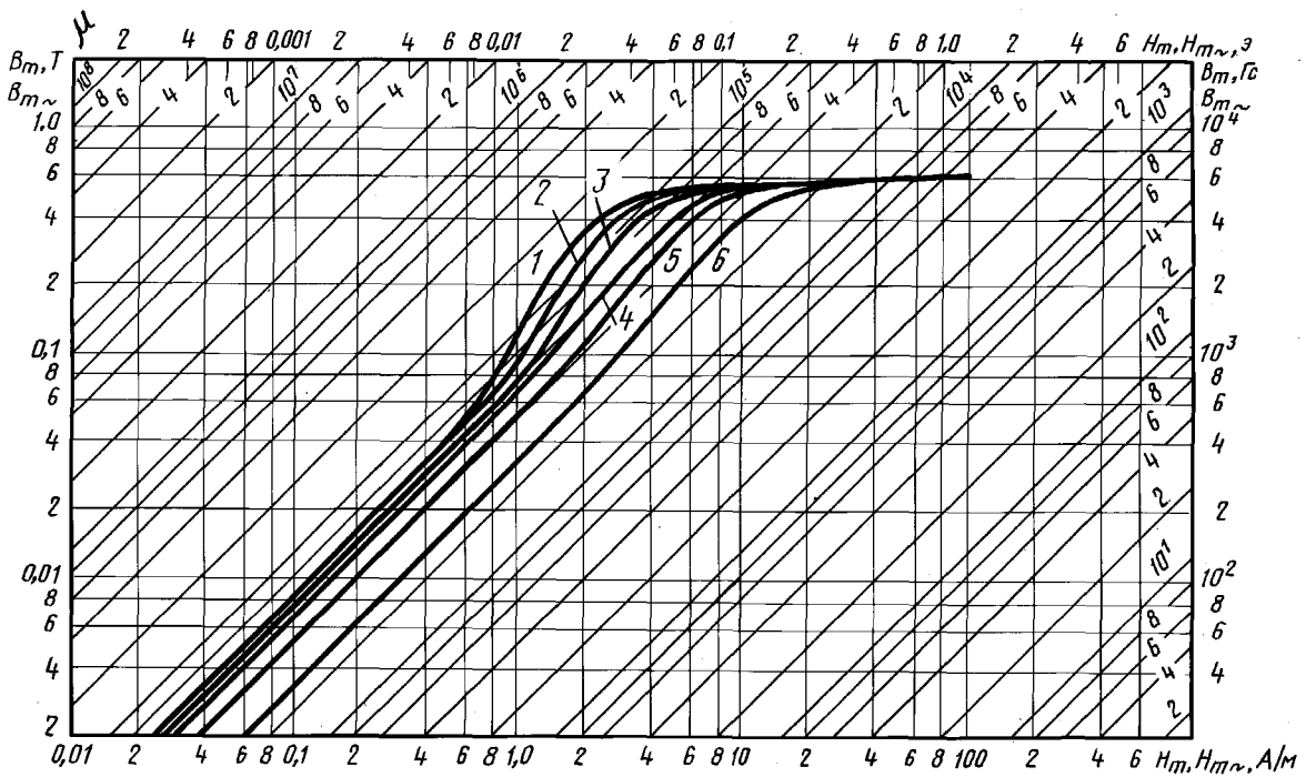
Кривые намагничивания сплава марки 83НФ толщиной 0,05 мм для частот: 1 — 0 Гц; 2 — 400 Гц; 3 — 1000 Гц; 4 — 2000 Гц; 5 — 4000 Гц; 6 — 10000 Гц
